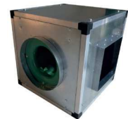
PFB - Plug-Fan Box Tamaño/Size 22 - 71 Max 22.875 m 3 /h - 5,5 kW
